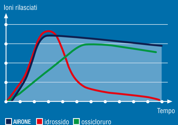
Rilascio ioni \text{Cu}^{++} nel tempo
